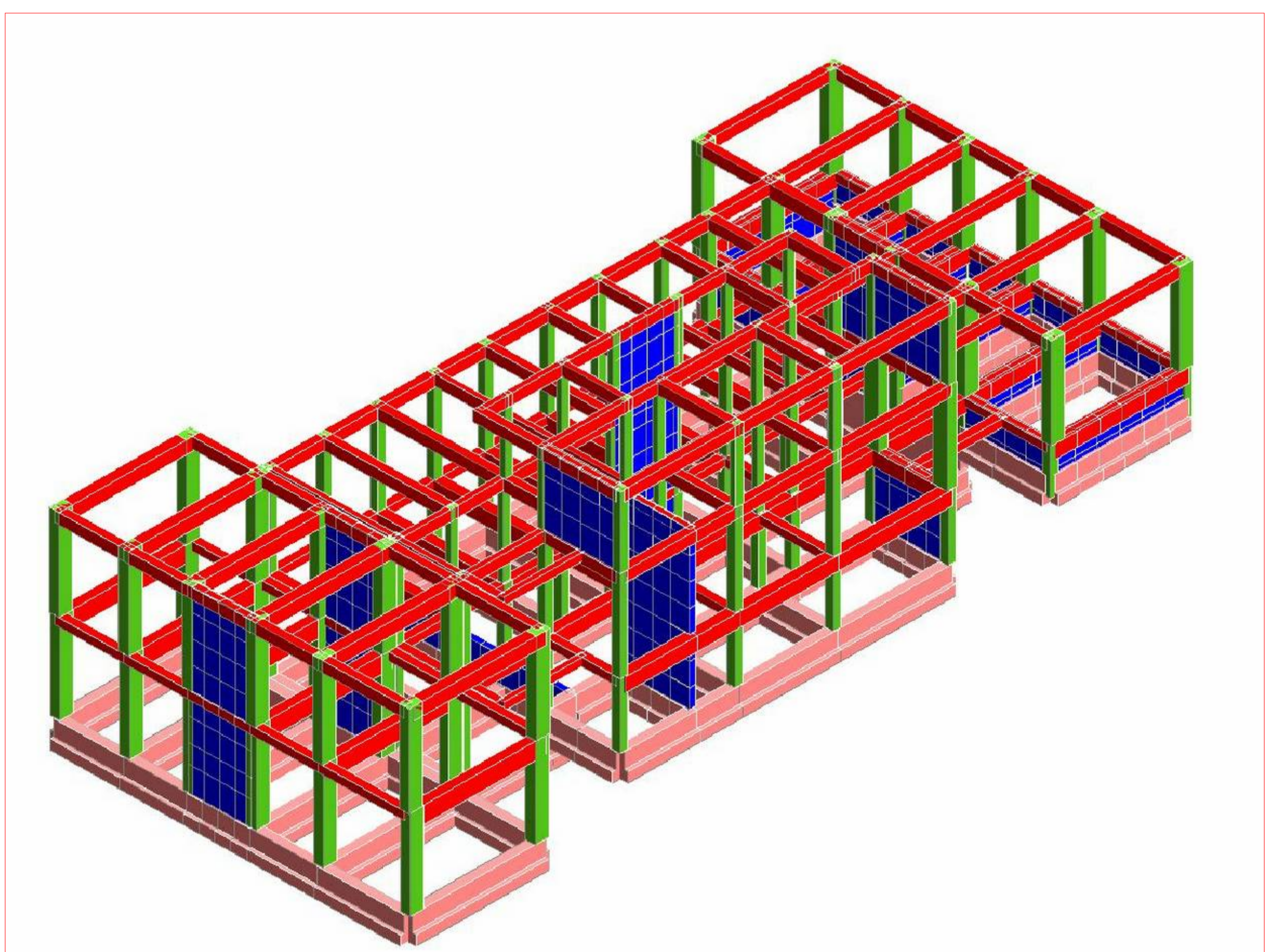
ASSONOMETRIA COMPLESSIVA
